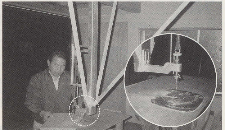
石島さんの使う糸鋸機にはアームがない
